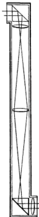
Рис. 97. Схема перископа подводной лодки.
